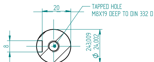
Przekrój A-A 1:1
